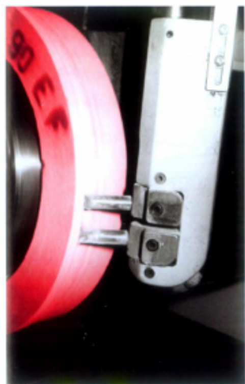
Diaform-Diamant- Meißel beim Profilieren einer kon- ventionellen Schleifscheibe (Bilder: Lach Dia- mant, Jakob Lach GmbH & Co. KG, Hanau)
