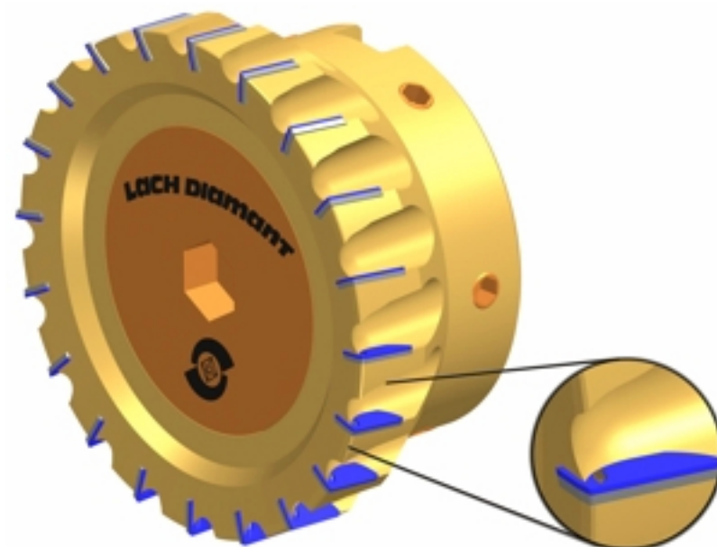
MB-X3 – Monoblock-PKD-Fräser für die Hochleistungszerspannung von Aluminium
