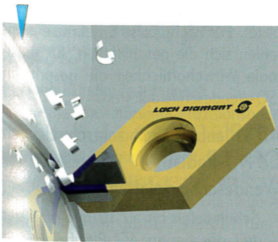
Dia-chipbreaker Type IC mit aktivem Spanbrecher und positivem Schnitt ab 0,1 mm Zustelltiefe.
