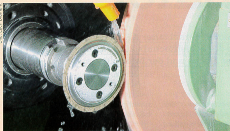
Drebojet-plus: Diamantrolle für das bahngesteuerte Abrichten und Profilieren von Schleifscheiben.
