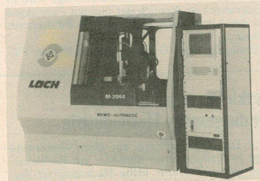
Diamant-Schleifmaschine mit ‚M-2050-Memo-Automatic‘
