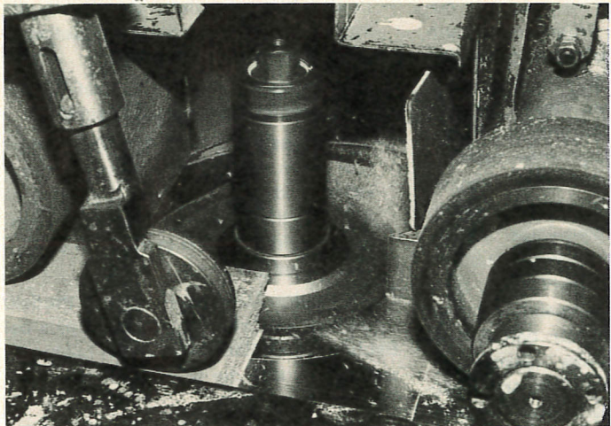
Lach-Spezial-Diamant-Nuter beim Fräsen eines Türfutters.
