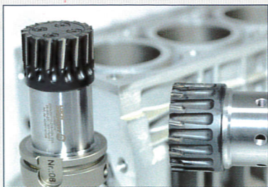
Heutige Hightech-Hochleistungs-Monoblockfräser mit extrem hoher Zähnezahl bis \varnothing 100 mm für die Aluminium-Motorfertigung – mit »Cool Injection« und Spanabweiser »Plus«.
