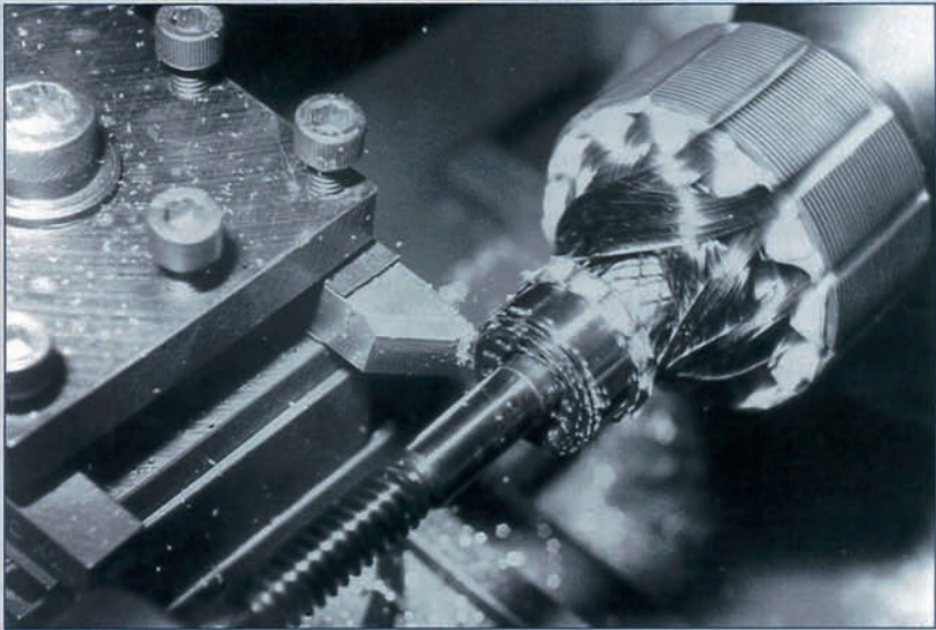
1973 – der Beginn der ersten Erfolgsstory durch PKD – wirtschaftlichere Kupfer-Kollektoren-Bearbeitung.
