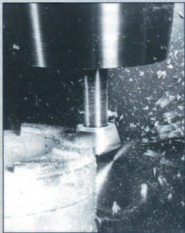
1974 LACH DIAMANT demonstriert auf der Hannover Frühjahrsmesse erstmals das Fräsen mit PKD von Kunststoffen und Aluminium (im Bild Zerspanung von GFK).
