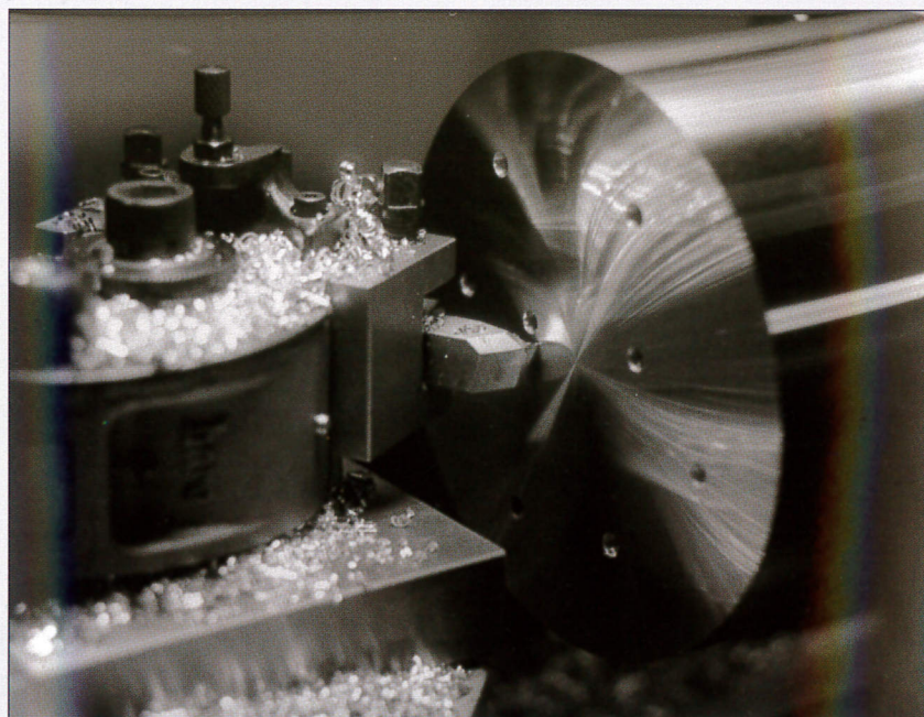
PKD-Drehwerkzeuge dreborid erstmals vorgestellt für hartmetall-überlegenes Drehen von Aluminium auf der Hannover Messe 1973.
