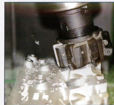
Erstmals Fräsen von Aluminium mit PKD-Fräsern auf der Hannover Messe 1974.
