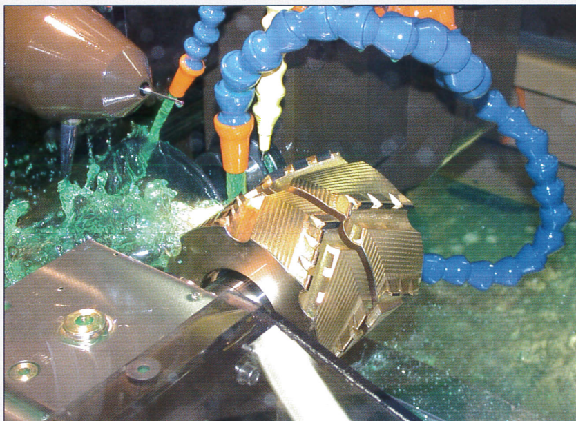
Funkenschleifen EDG-plus auf einer LACH-Universal-Schärfmaschine.
