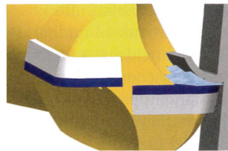
Kühlt direkt an der Schneide: der PKD-Monoblock-Fräser
