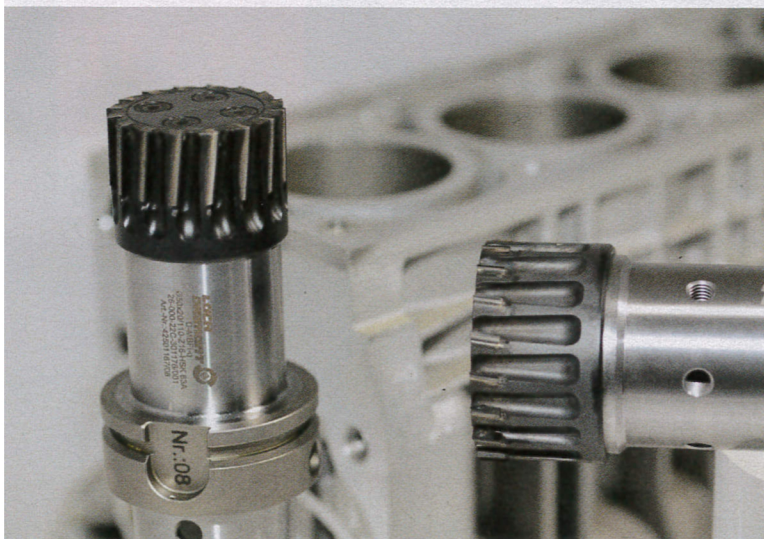
»Cool Injection-Plus« mit Kühlung direkt und Spanabweiser.
