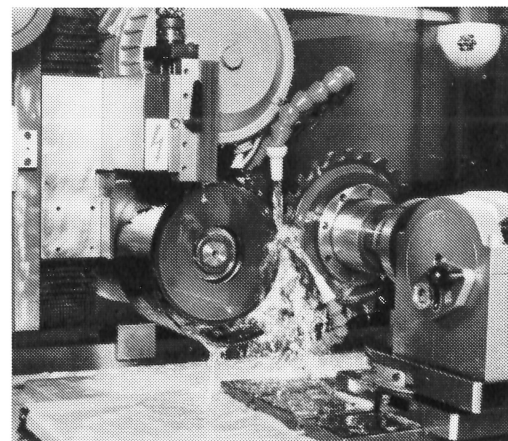
Abbildung 2 Schleifen eines Diamant-Zerspaners
