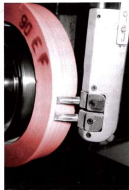
Bild 2: Diaform-Diamant-Meißel beim Profilieren einer konventionellen Schleifscheibe (Werkbilder: Lach Diamant Jakob Lach GmbH & Co. KG, Hanau)
