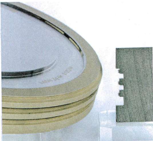
Profilschleifscheibe mit Bindung Spezial-Metall CX5 Ø 150 x 15 mm für HM-Gewindeschleifen (im Bild mit Prüfschablone)
